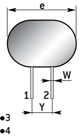
Sorties radiales Modèle PM 89 R enrobé
